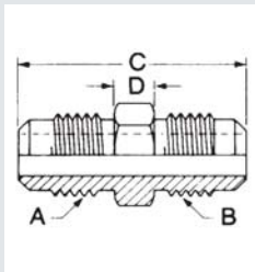
Union- Flare to Flare
