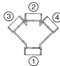
DWV 45° Double Y
